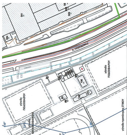
ΠΕΡΙΟΧΗ Δ_ΚΑΙΜΑΚΑ 1:200
